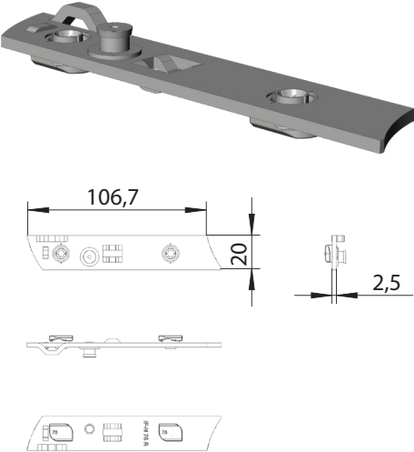
Z0110006188-K05 - Rahmenanbindung RA.DB.A.IF-N.78.RS
