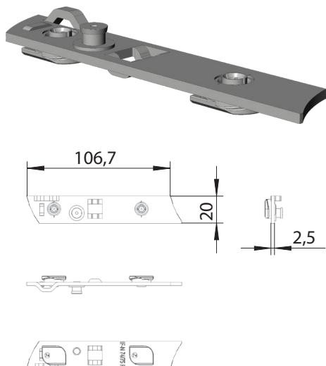
Z0110006188-K01 - Rahmenanbindung RA.DB.A.IF-N.74.RS
