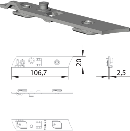
Z0110006188-K04 - Rahmenanbindung RA.DB.A.IF-N.75.LS
